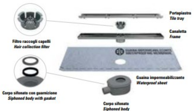
Il porta piastrella è dotato di fermi in gomma The tile holder is equipped with rubber stops
