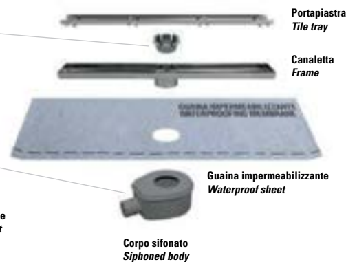
Corpo sifonato con guarnizione Siphoned body with gasket
