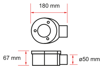
Corpo sifonato/Drain body
